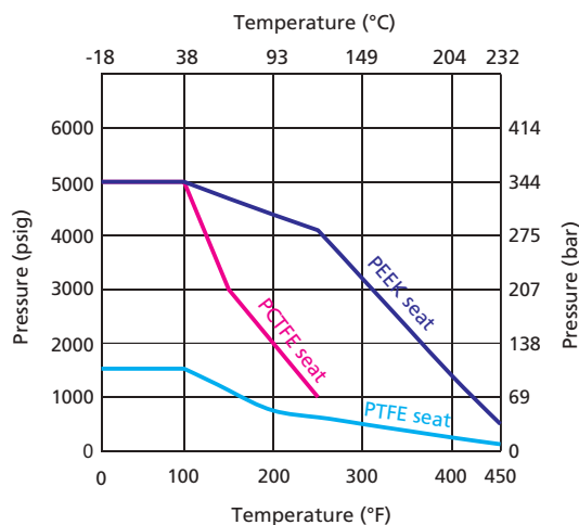
Alloy 400 Body
